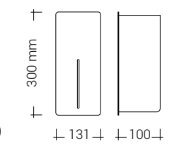
LOKI SEIFEN-/DESINFIZIATIONSMITTELSPENDER
